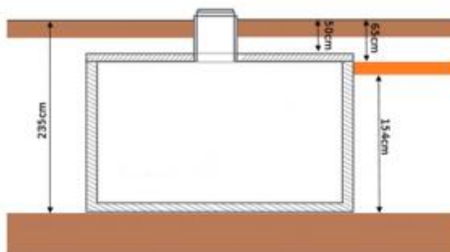
RYSUNEK 5: SCHEMAT GŁĘBOKOŚCI POSADOWIENIA ZBIORNIKA 10M 3
