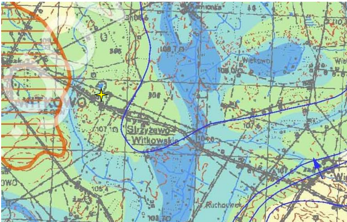
RYСУNEK 10: LOKALIZACJA INWESTYCJI WZGLĘDEM GŁĘBOKOŚCI DO PIERWSZEGO POZIOMU WODONOŚNEGO
